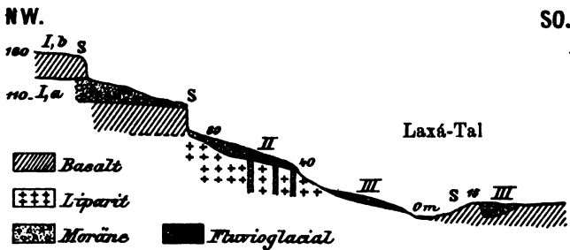
Fig. 3. Profil durch das Laxá-Tal. I., II., III. Gebilde dreier Eiszeiten; S = Glazialschrammen.
